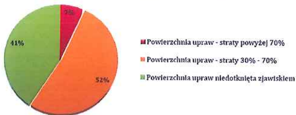
Gmina Trzemeszno - susza 2018
