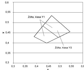
Rys. 2. Współrzędne chromatyczności x,y dla barwy żółtej oznakowania
