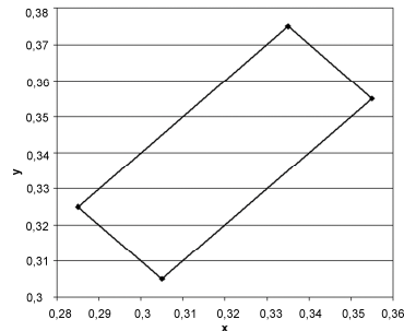
Rys. 1. Współrzędne chromatyczności x,y dla barwy białej oznakowania
