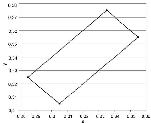
Rys. 1. Współrzędne chromatycyjnosc x,y dla barwy bialej oznakowania
