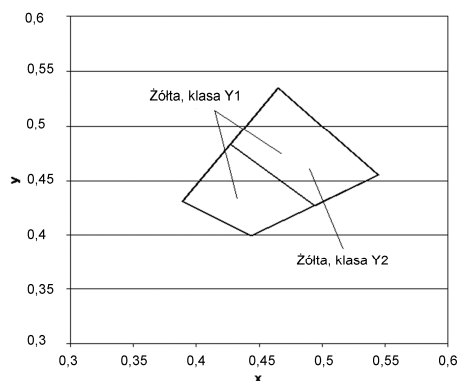
Rys.2. Współrzędne chromatycyjnosc x,y dla barwy zoltej oznakowania
