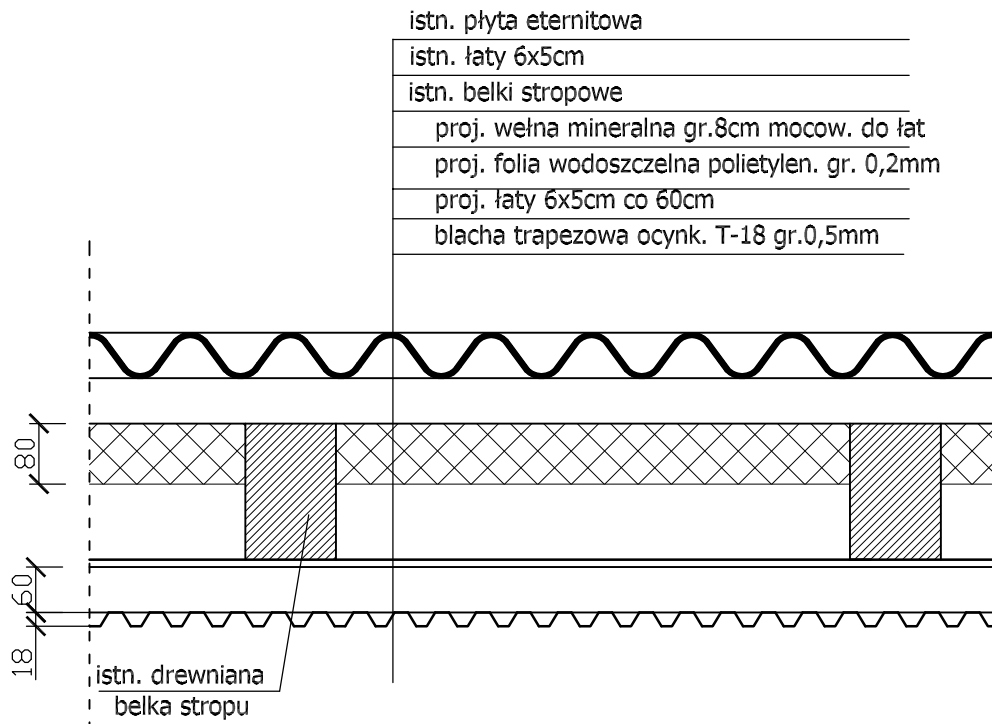
Przekrój poprzeczny 1:10
