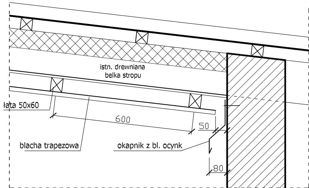
Detail okapnika 1:10
