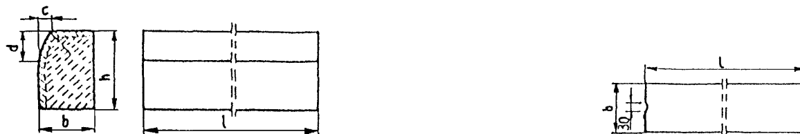
Rys. 1. Wymiarowanie krawężników
