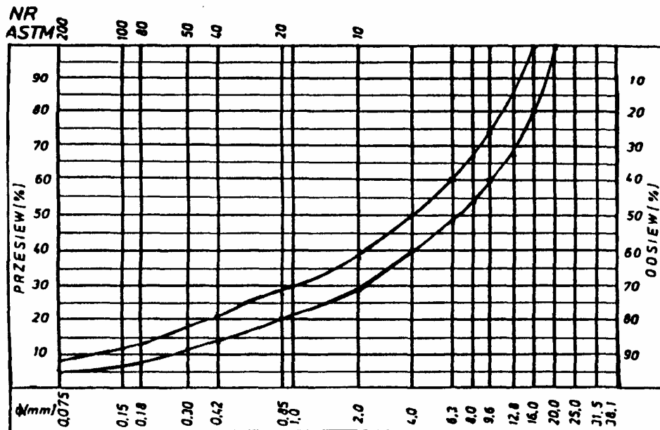
Rys. 4. Krzywe graniczne uziarnienia mieszanki mineralnej 0+20 mm do warstwy ściernalnej z betonu asfaltowego dla KR 3-6
